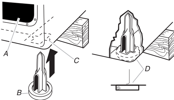
A. Panneau arrière de la laveuse B. Pied de nivellement arrière C. Trou en bas de la laveuse pour pied de nivellement arrière D. Pied de nivellement arrière enfoncé en bas de la laveuse
