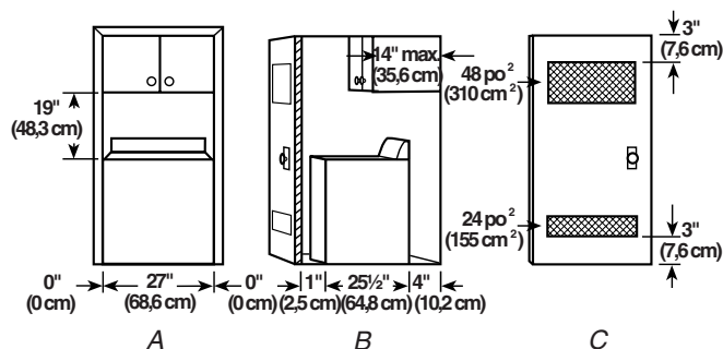
A. Vue avant B. Vue de profil C. Porte de placard avec ouvertures d'aération
