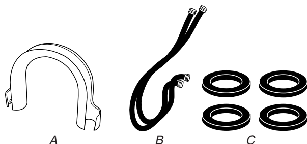
A. Bride de retenue du tuyau de vidange B. Tuyaux d'arrivée d'eau (2) C. Joints plats pour les raccords des tuyaux d'eau (4)
